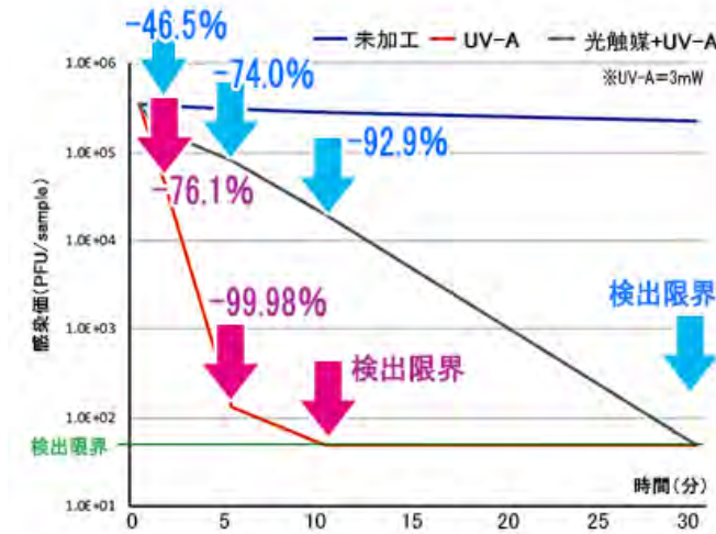
図1 UV-A照射によるウイルス除去の推移
